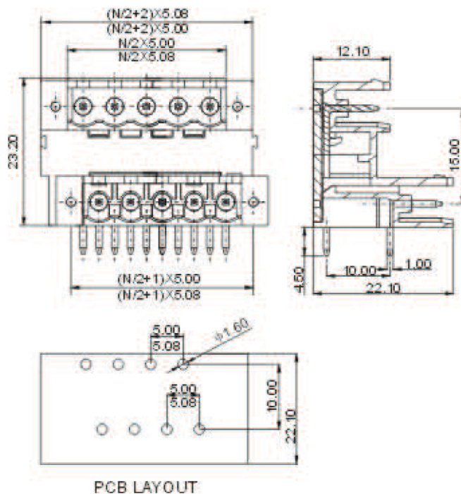
2EDGRTM-5.0 2EDGRTM-5.08
